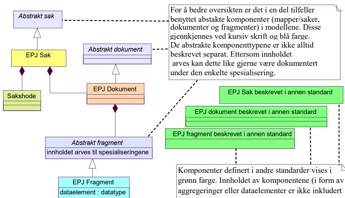
Figur 22 Symboler for komponenttyper
