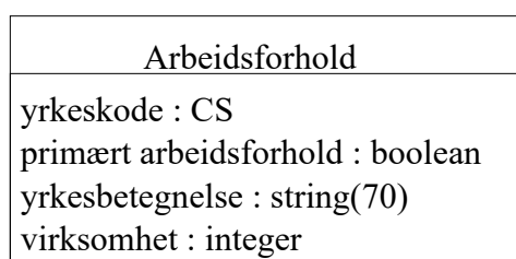
Figur 16 Eksempel på klasse med attributter
